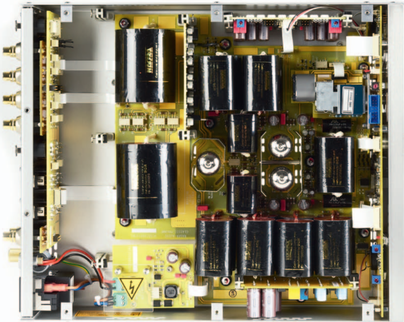
Voluminöse Folienkondensatoren dominieren die mit vergoldeten Leiterbahnen versehene Printplatte des Vorverstärkers, der von einem unscheinbaren Schaltnetzteil (links unten hinter der Netzbuchse) versorgt wird. Hinter dem Anschlussfeld bleibt Platz frei für optionale Ein- und Ausgangsübertrager. Die drei Doppeltrioden sind mit Abschirmblechen umgeben, als Pegelsteller dient ein motorisierter ALPS-Poti.
